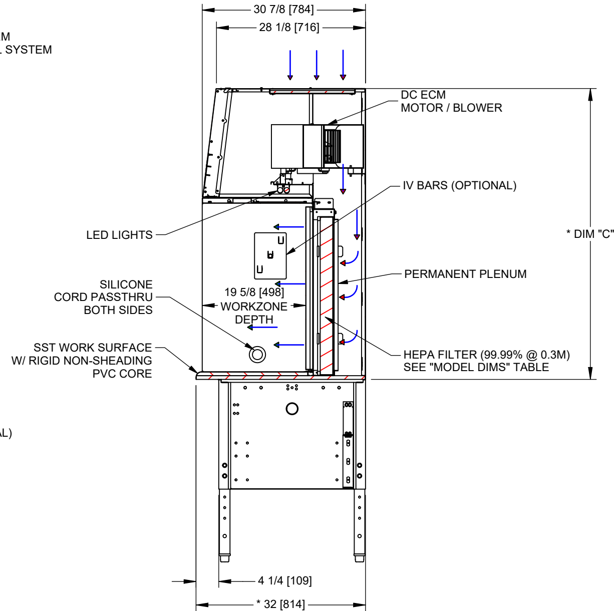
SECTION A-A
